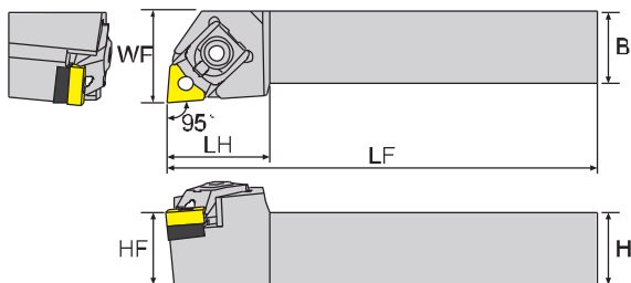
寸法 Dimension(mm)
